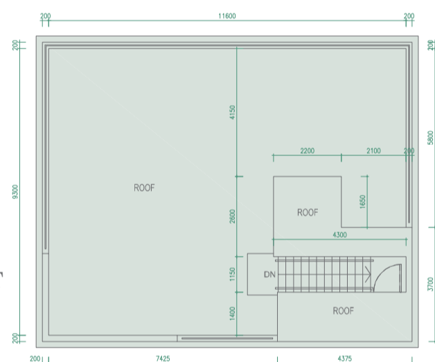
Floor Plan R/F 天台平面圖
