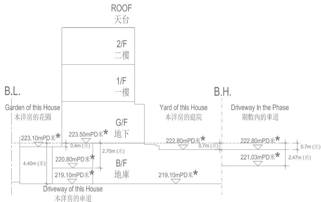
Section A 剖面圖 A
