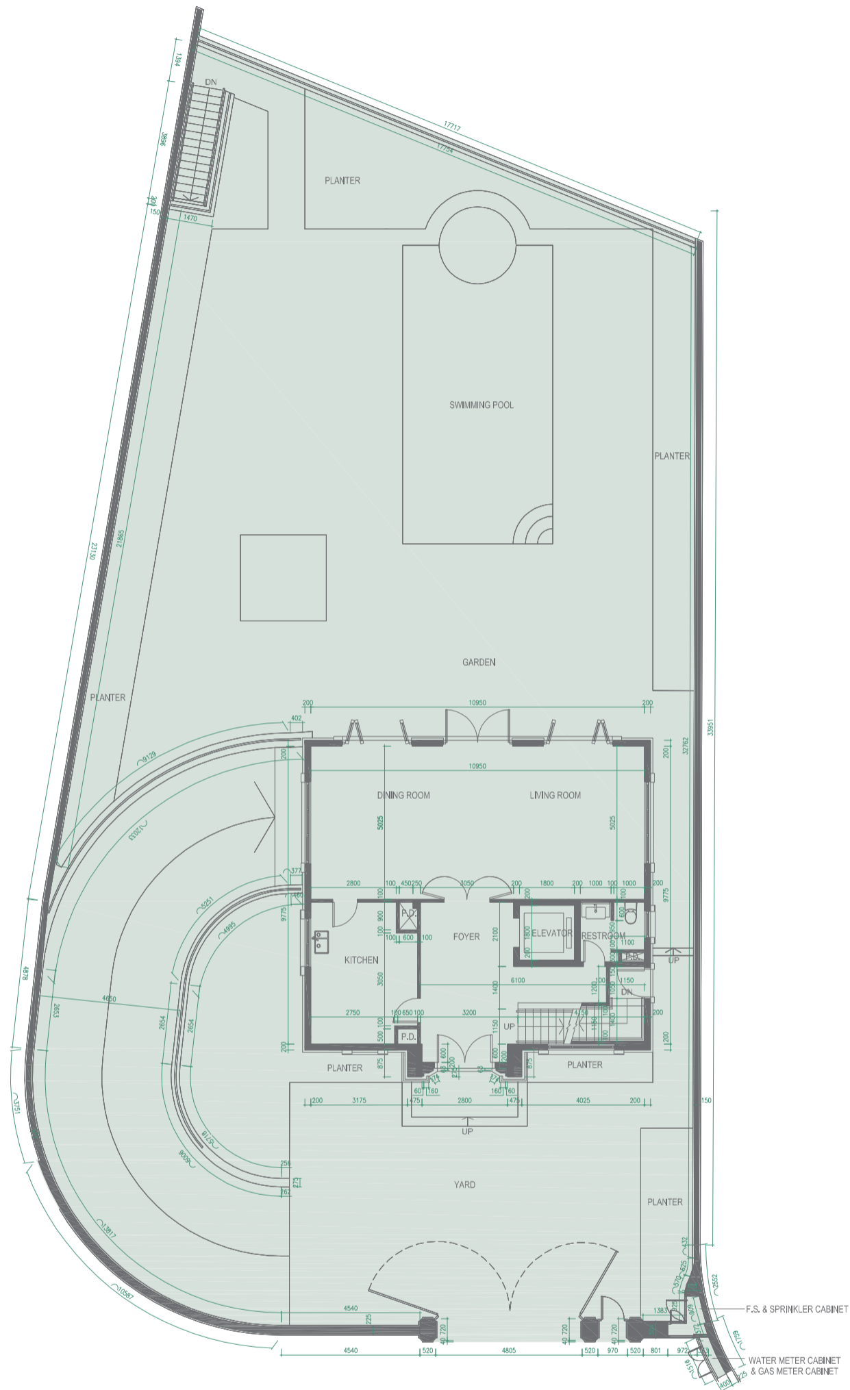
Floor Plan G/F 地下平面圖
