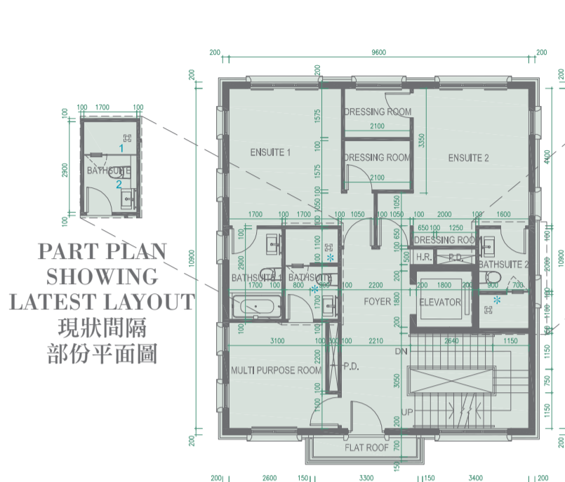
Floor Plan 1/F 一樓平面圖
