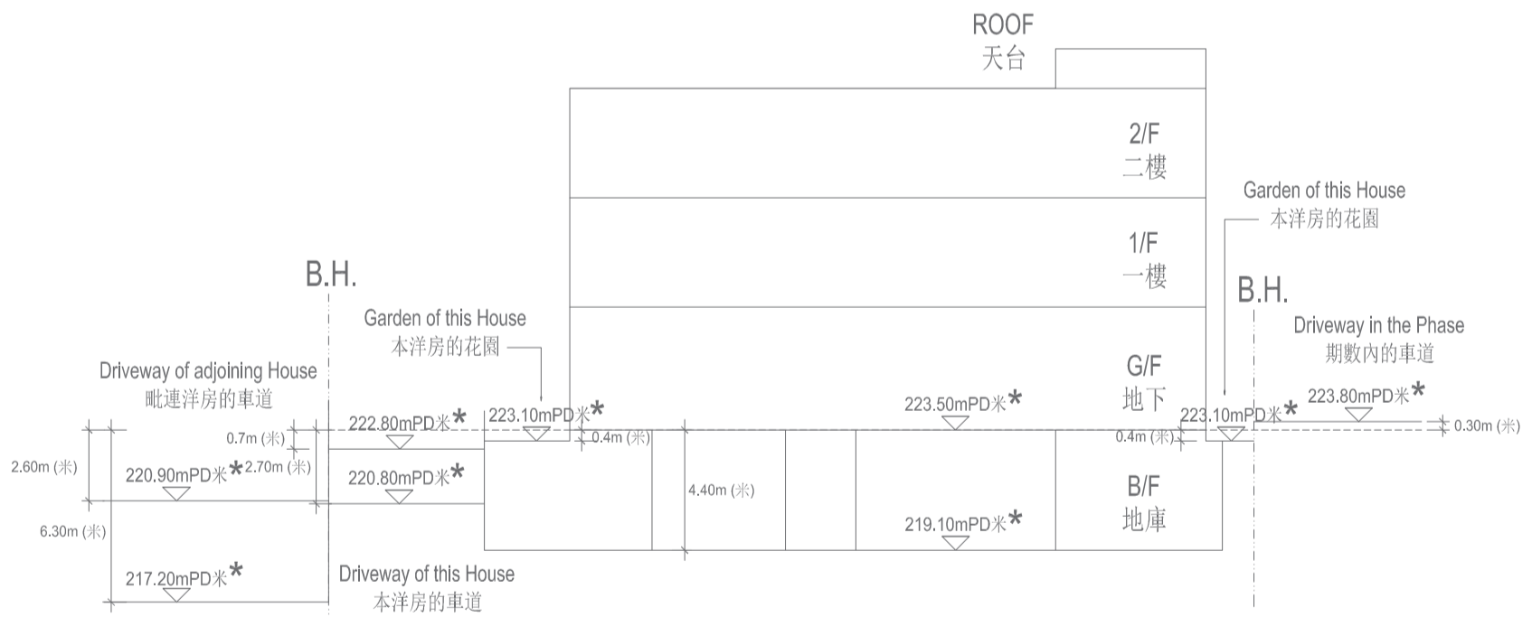
Section B 剖面圖 B
