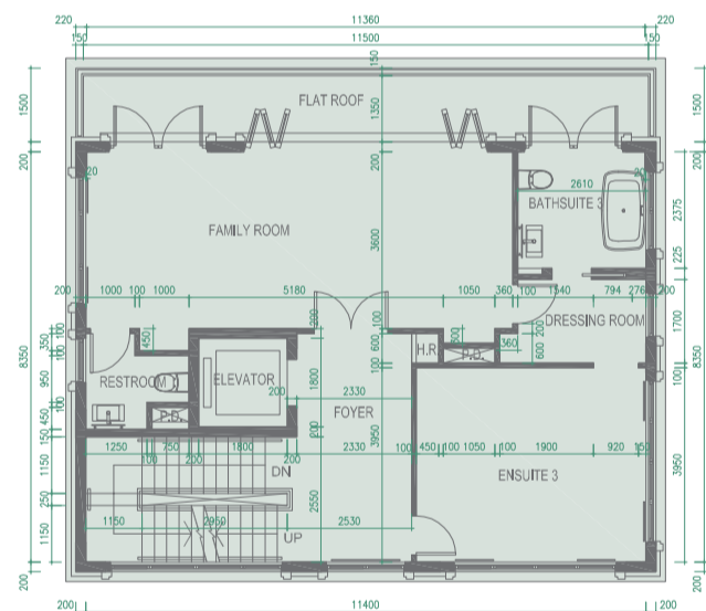
Floor Plan 3/F 三樓平面圖
