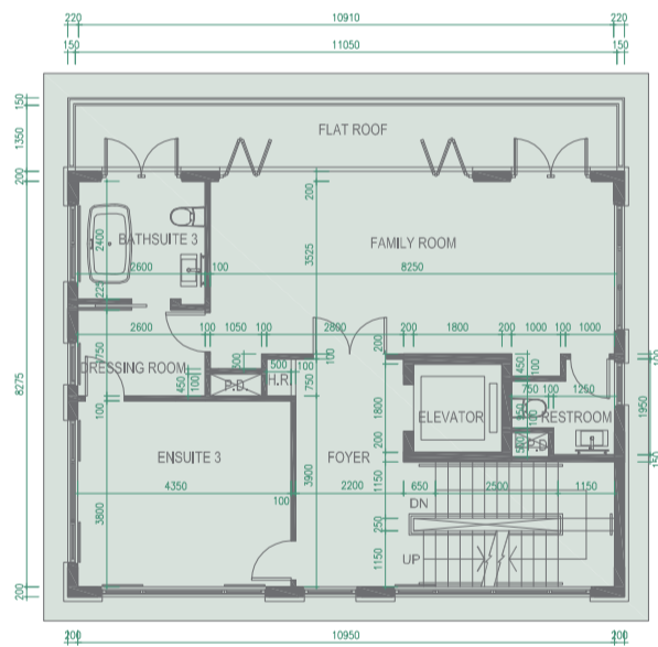
Floor Plan 3/F 三樓平面圖
