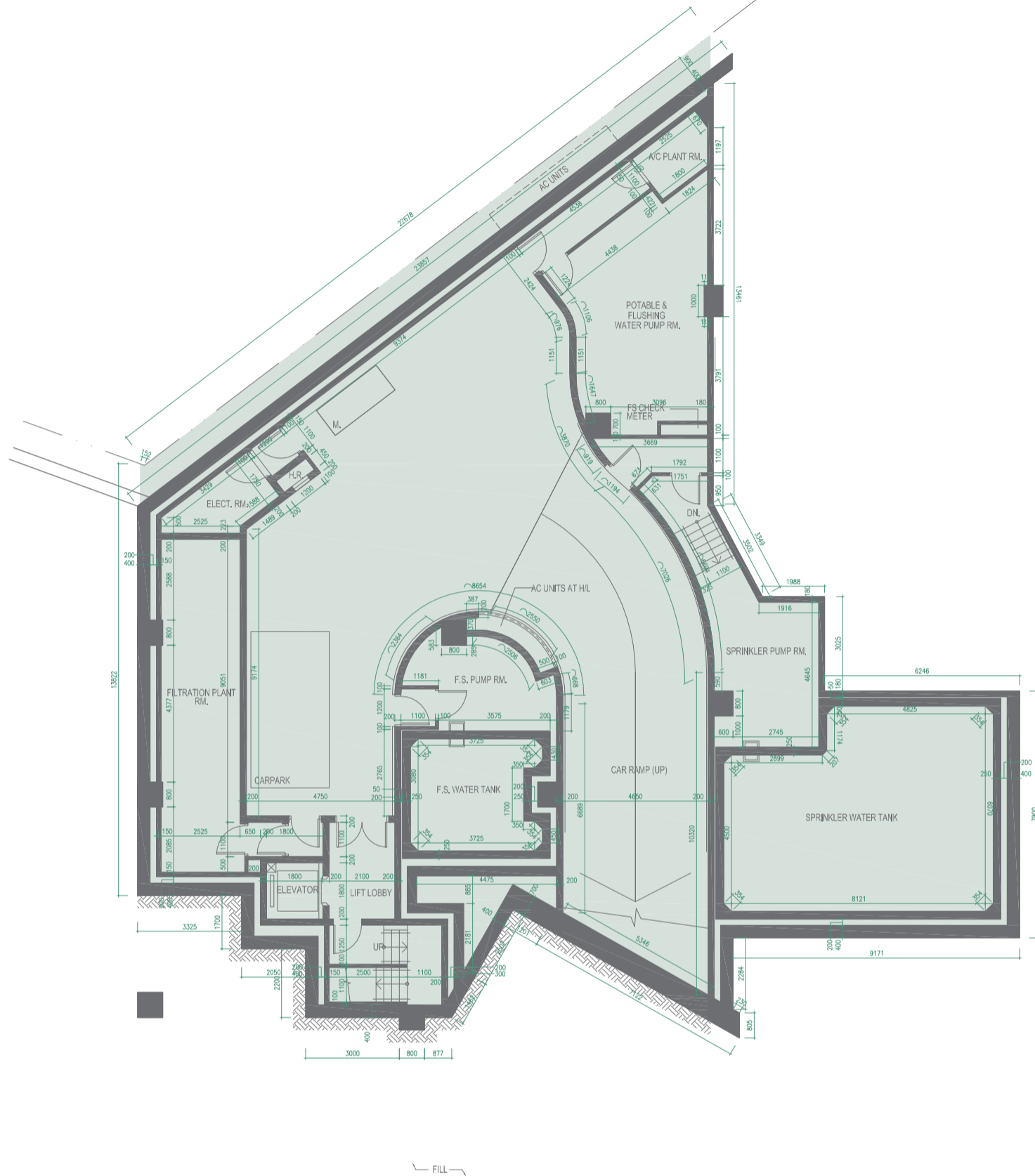
Floor Plan B/F 地庫平面圖
