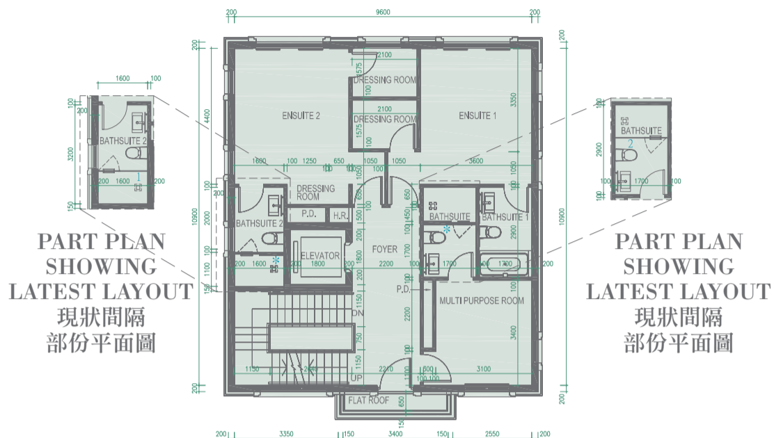
Floor Plan 1/F 一樓平面圖
