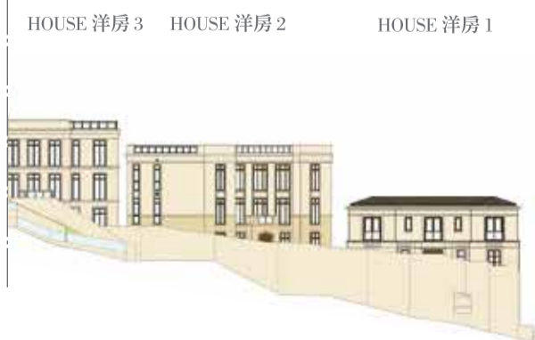
Elevation 4 立面圖四
