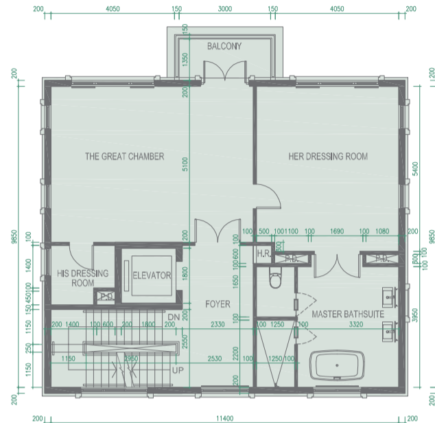
Floor Plan 2/F 二樓平面圖
