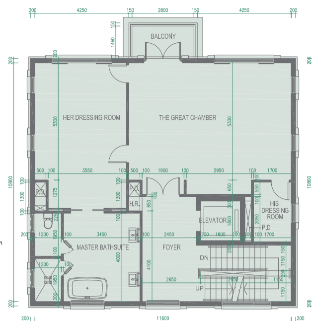
Floor Plan 2/F 二樓平面圖
