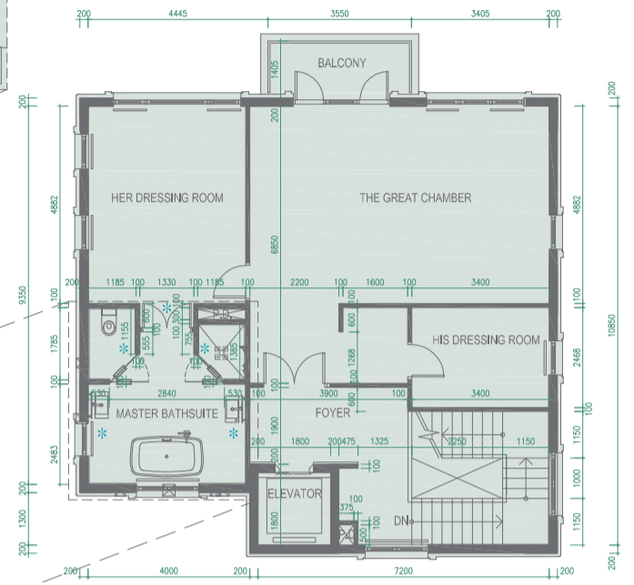
Floor Plan 2/F 二樓平面圖
