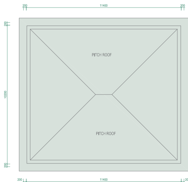
Floor Plan R/F 天台平面圖
