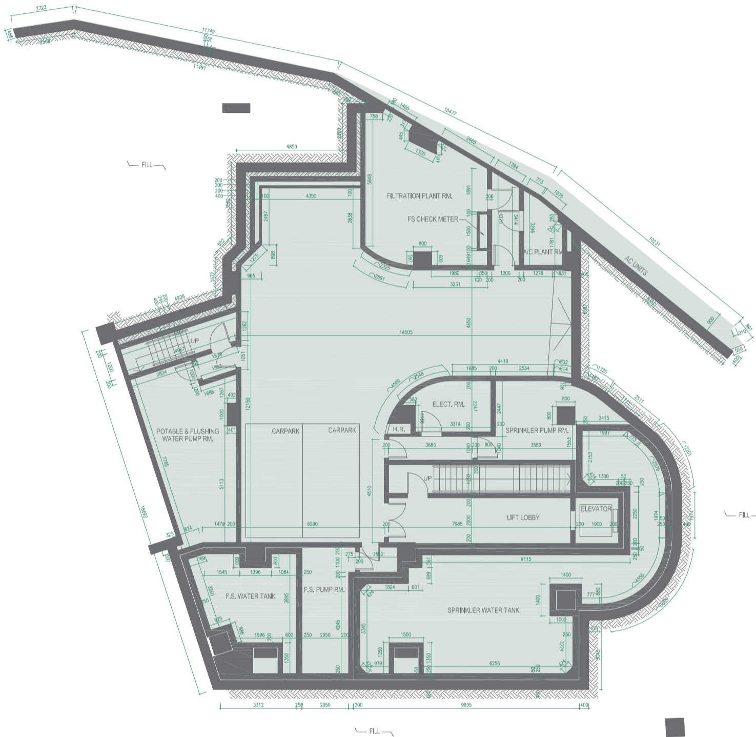
Floor Plan B/F 地庫平面圖
