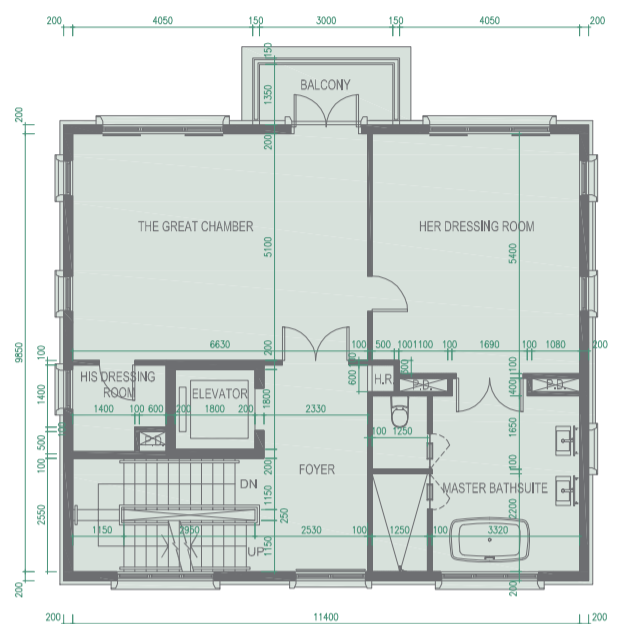
Floor Plan 2/F 二樓平面圖
