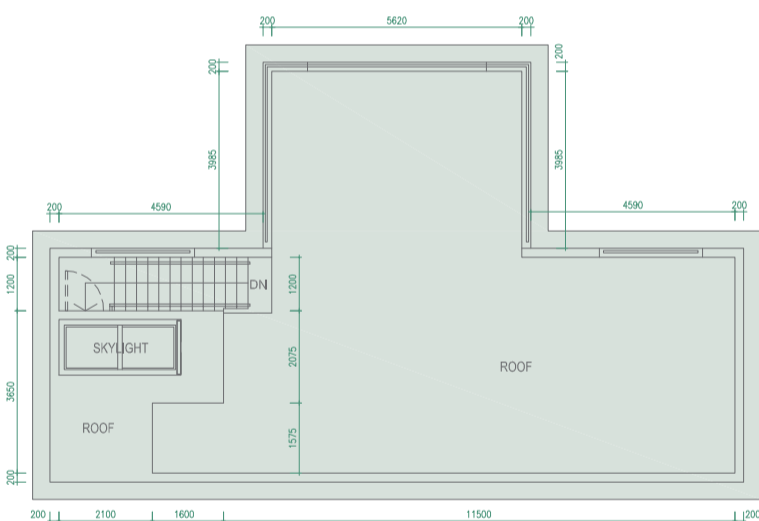
Floor Plan R/F 天台平面圖
