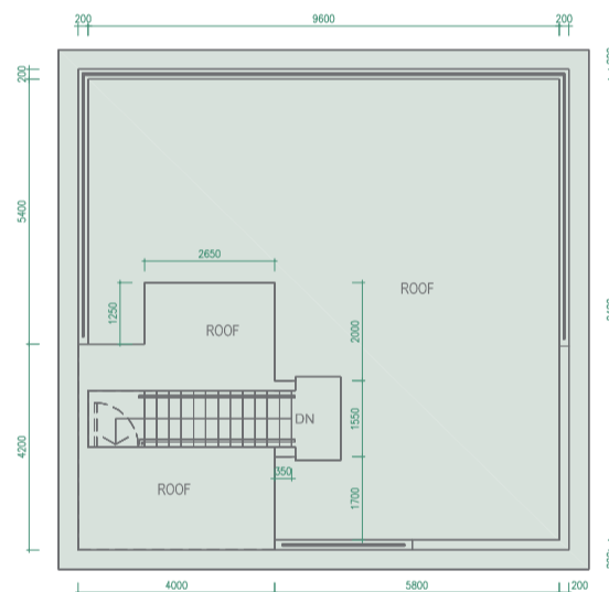
Floor Plan R/F 天台平面圖
