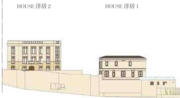
Elevation 2 立面圖二
