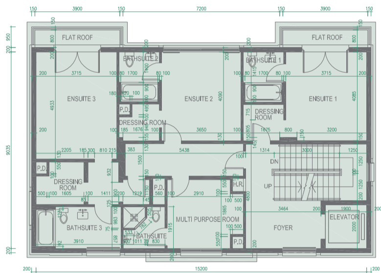
Floor Plan 1/F 一樓平面圖
